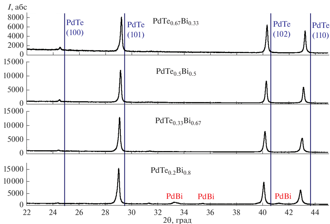
Рис. 1. Фрагменты рентгенограмм образцов \text{PdTe}_{1-x}\text{Bi}_x ( x = 0.33, 0.5, 0.67, 0.8 ): смещение отражений фаз \text{PdTe}_{1-x}\text{Bi}_x относительно отражений чистого PdTe.
