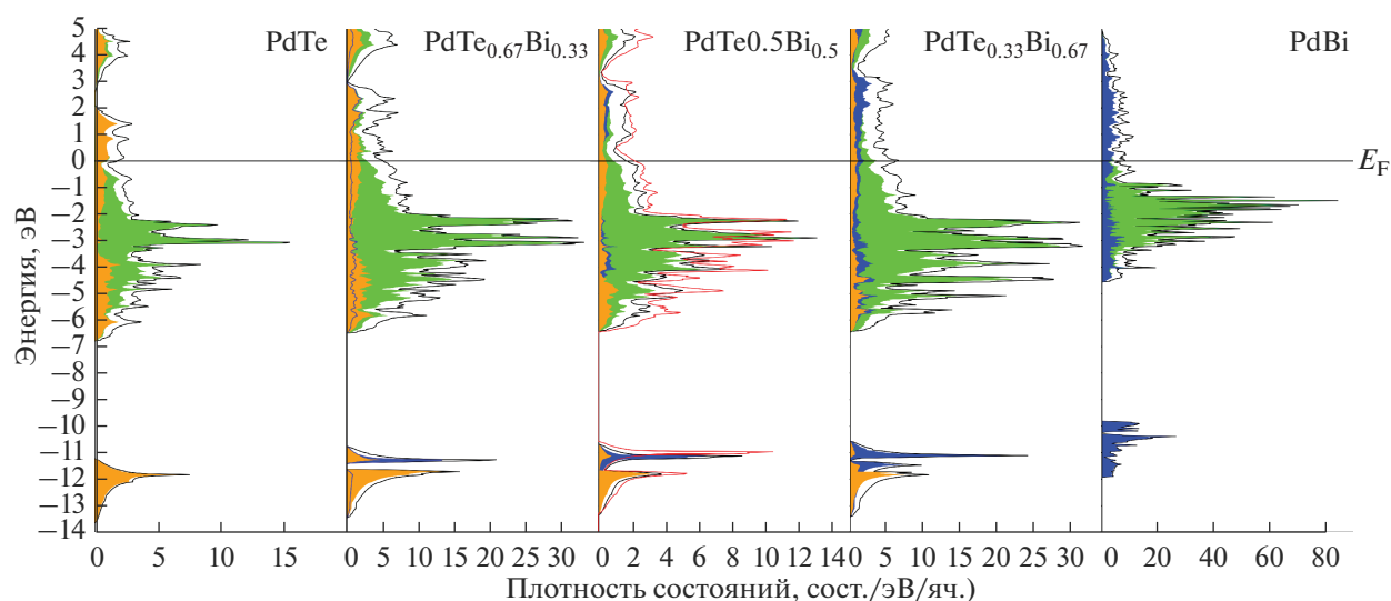
Рис. 5. Общая и парциальная плотность состояний вблизи уровня Ферми для PdTe, PdTe 1-x Bi x ( x = 0.33, 0.5, 0.67 ) и PdBi. Вклады Pd показаны зеленым, Te — оранжевым, Bi — синим, общая плотность — черной линией. Красная линия для PdTe 0.5 Bi 0.5 показывает общую плотность состояний для расчета с учетом спин-орбитального взаимодействия.
