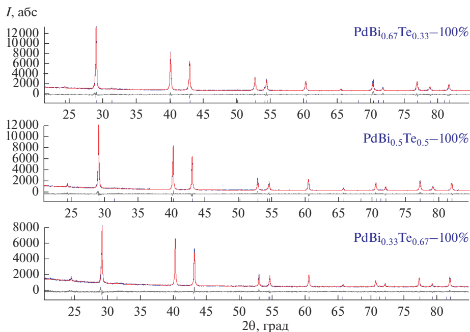
Рис. 2. Экспериментальные, расчетные и разностные рентгенограммы для однофазных образцов \text{PdTe}_{1-x}\text{Bi}_x ( x = 0.33, 0.5, 0.67 ).
