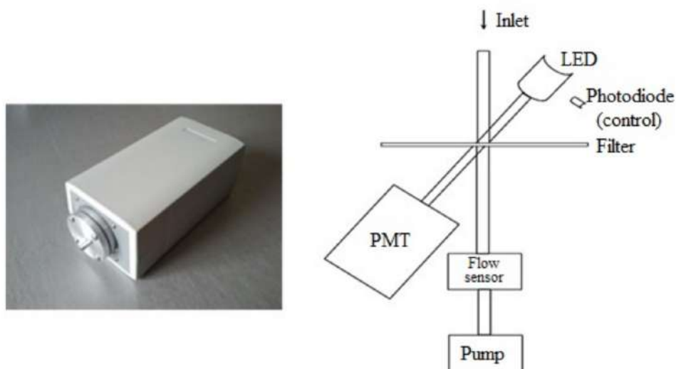
Рис. 2.1.1.2. Портаэталометр-A1 и схема его устройства
