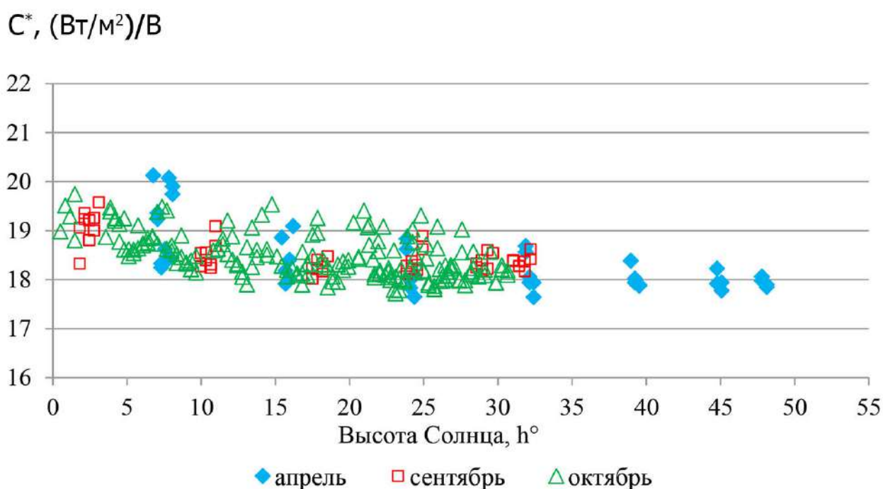
Рисунок 1.3.2.1. Переводные множители прибора UVA-1 YES №060902 (контрольный), отградуированного по прибору UV-S-A-T фирмы Kirr&Zonen №110062 с использованием градуировки, полученной в Давосе. Пасмурное небо. (апрель – до градуировки, сентябрь-октябрь – после градуировки)
