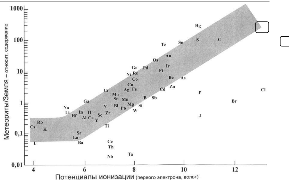
Рис. 4. Сравнительная распространённость элементов в зависимости от потенциалов ионизации в поясе астероидов относительно Земли
