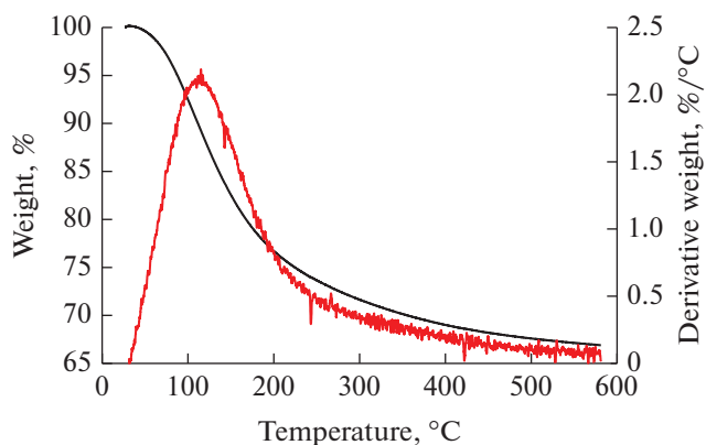
Рис. 5. Кривая ДТГ образца НОАМ-2h.
