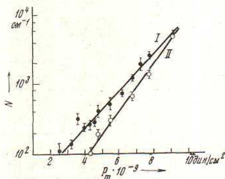
Рис. 2. Зависимости плотности дислокаций N от величины максимального нормального напряжения P_m , полученные при микродеформации LiF на воздухе (I) и в вазелиновом масле (II). Усреднение по 120 образцам
