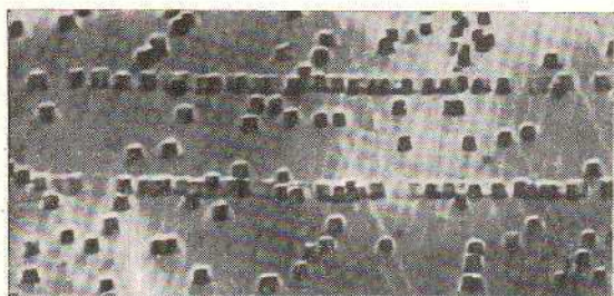
Рис. 1. Дислокационная структура, возникающая в процессе скольжения индентора по поверхности LiF на воздухе при силе поджима F = 15 дин. 125\times
